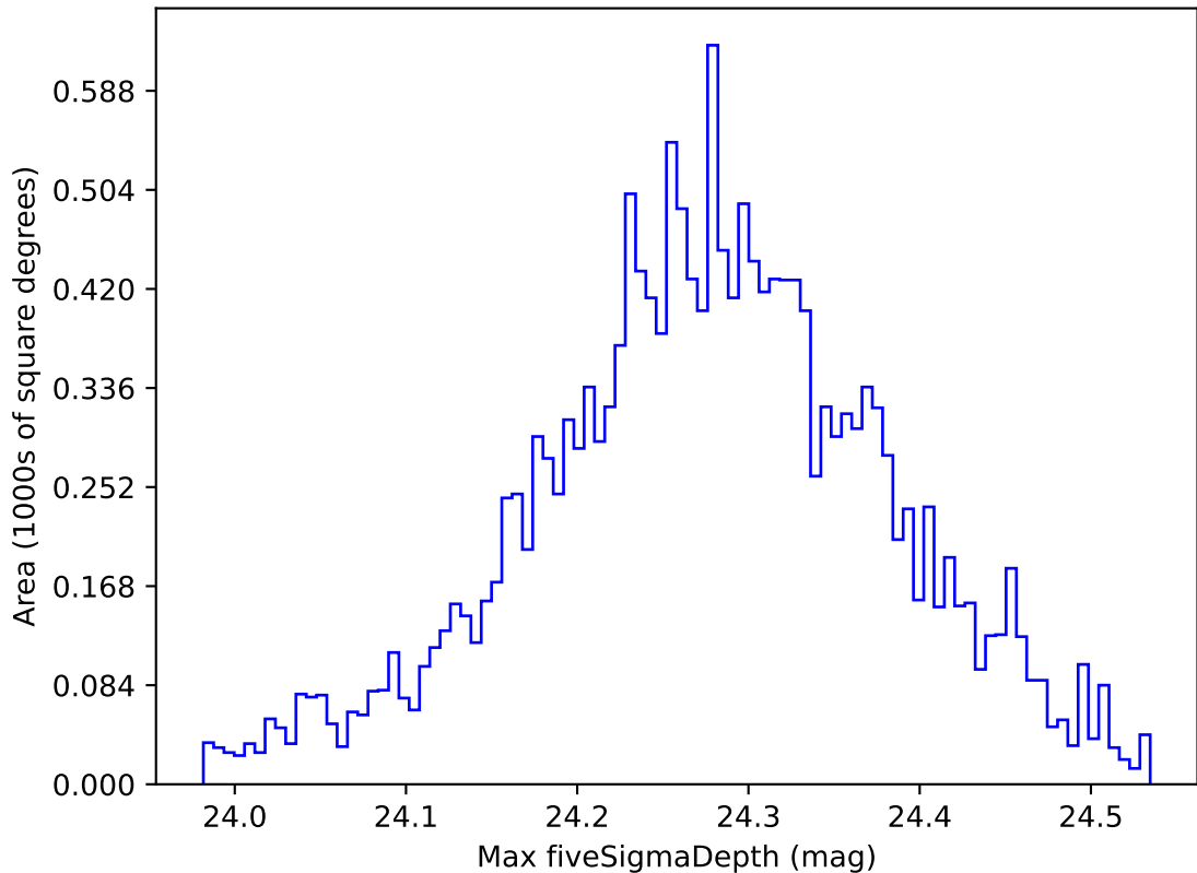
weather_cloudso20v3.4_10yrs WFD i band: Max fiveSigmaDepth
