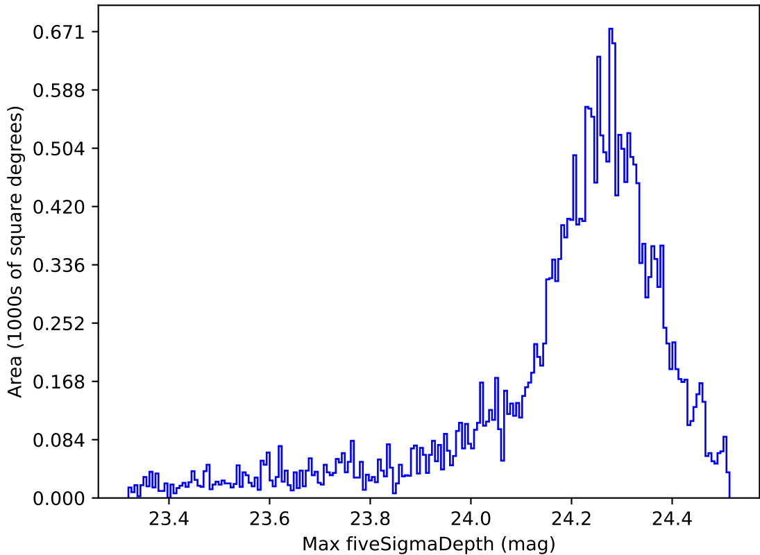
weather_cloudso20v3.4_10yrs All sky i band: Max fiveSigmaDepth
