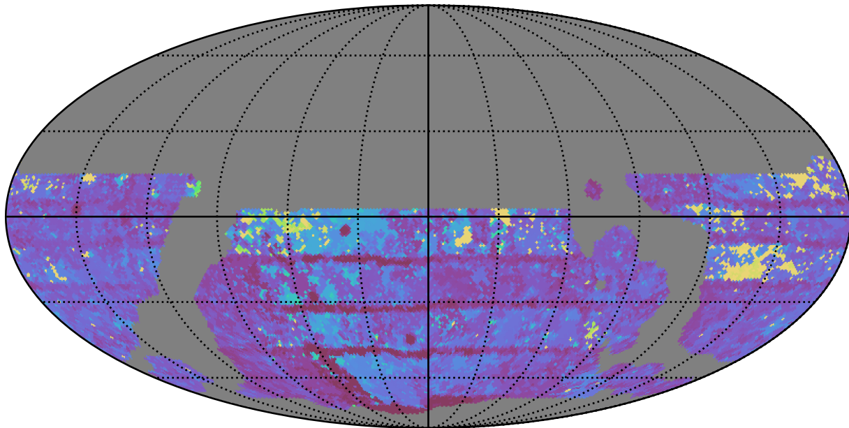
weather_cloudso20v3.4_10yrs WFD y band: Max Inter-Night Gap
