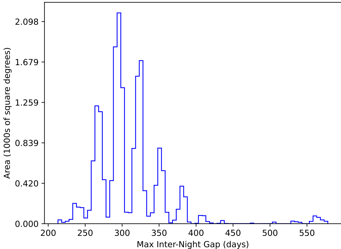
weather_cloudso20v3.4_10yrs WFD y band: Max Inter-Night Gap
