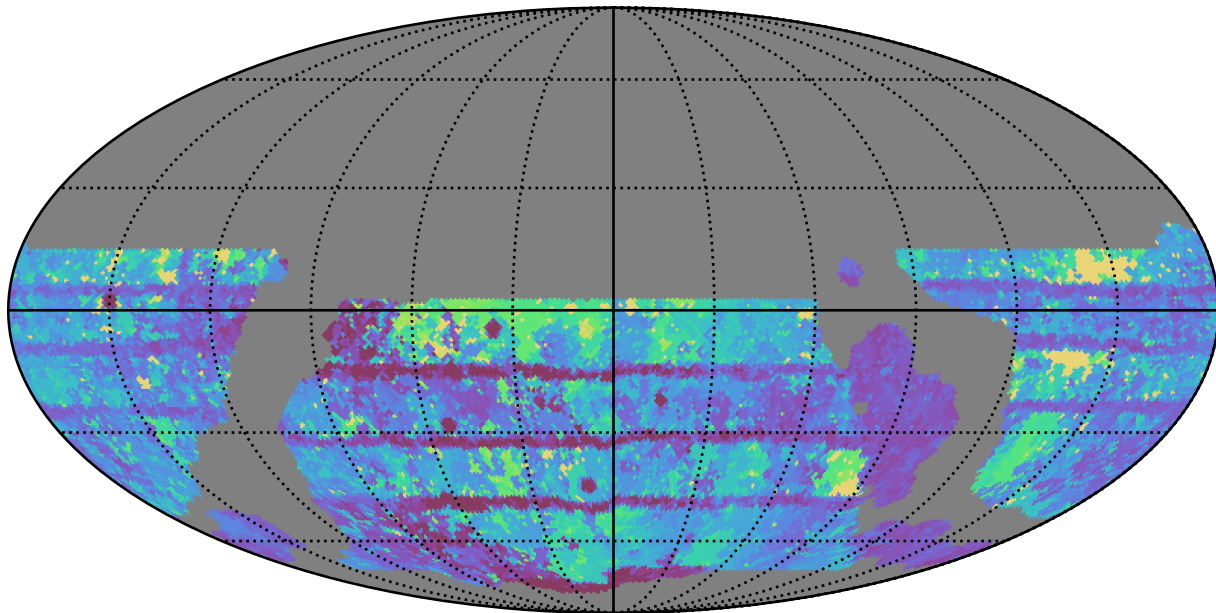
weather_cloudso20v3.4_10yrs WFD i band: Max Inter-Night Gap
