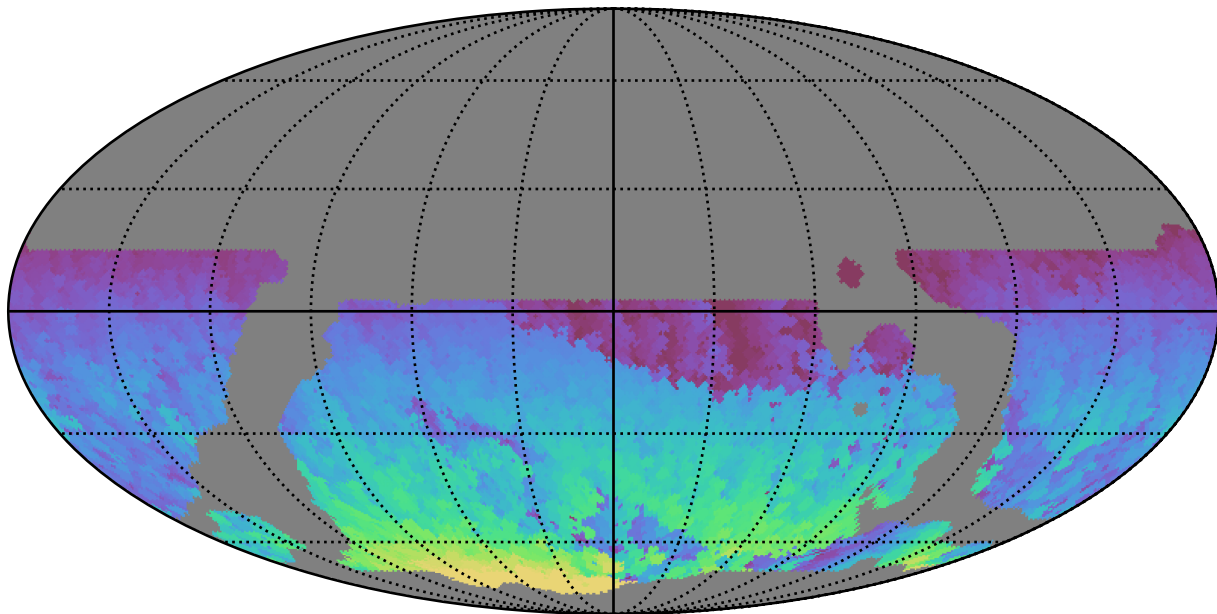
weather_cloudso20v3.4_10yrs WFD z band: Max HA
