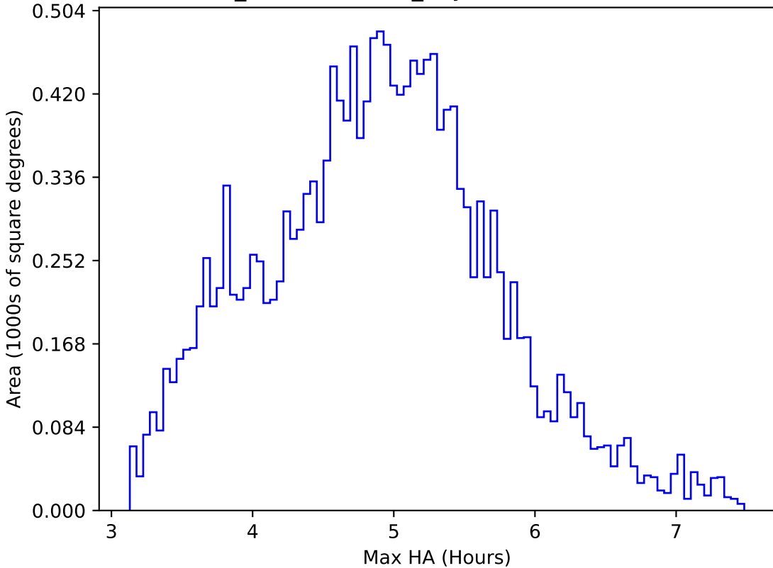
weather_cloudso20v3.4_10yrs WFD z band: Max HA
