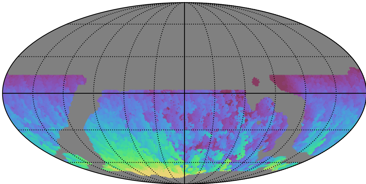
weather_cloudso20v3.4_10yrs WFD y band: Max HA
