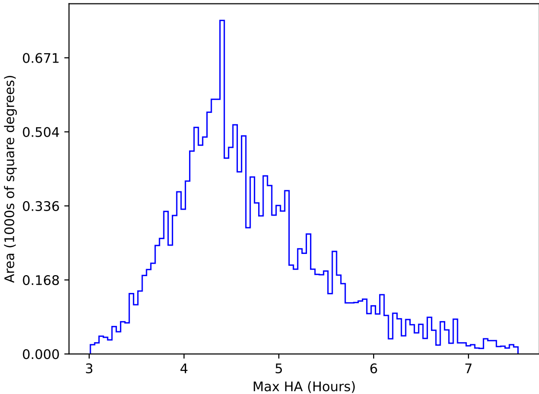
weather_cloudso20v3.4_10yrs WFD y band: Max HA
