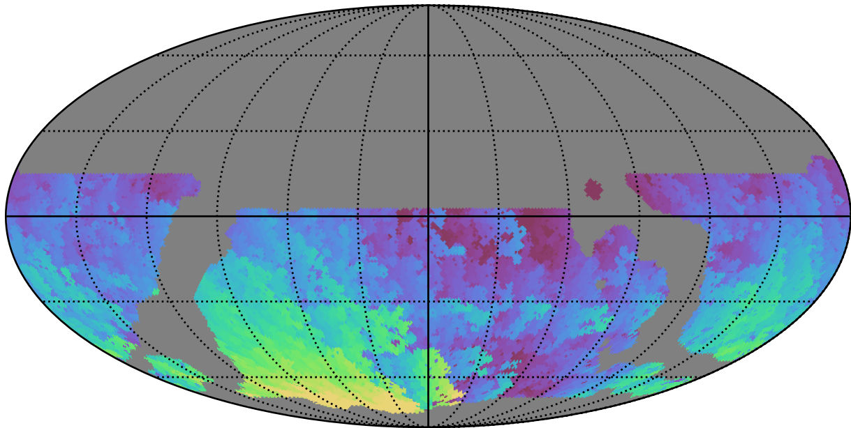
weather_cloudso20v3.4_10yrs WFD u band: Max HA
