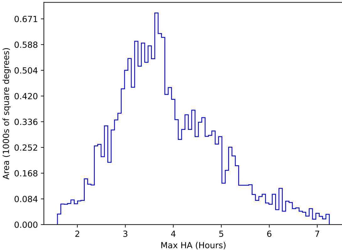
weather_cloudso20v3.4_10yrs WFD u band: Max HA
