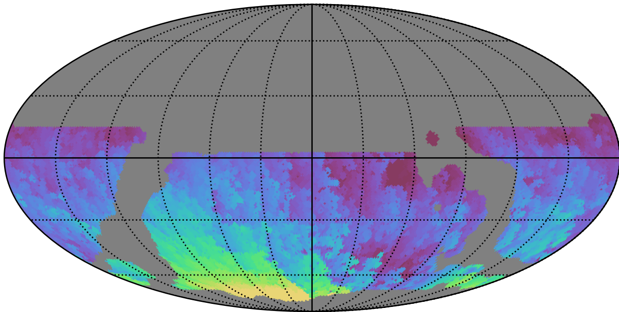
weather_cloudso20v3.4_10yrs WFD r band: Max HA
