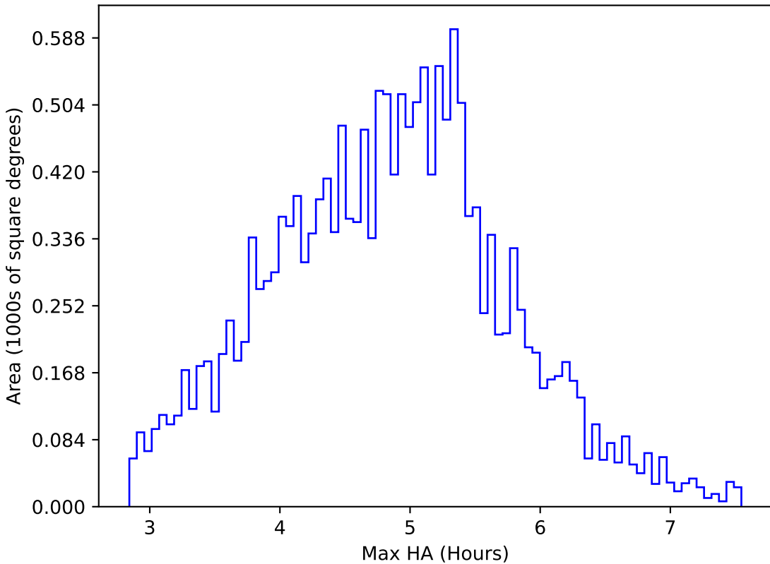
weather_cloudso20v3.4_10yrs WFD i band: Max HA
