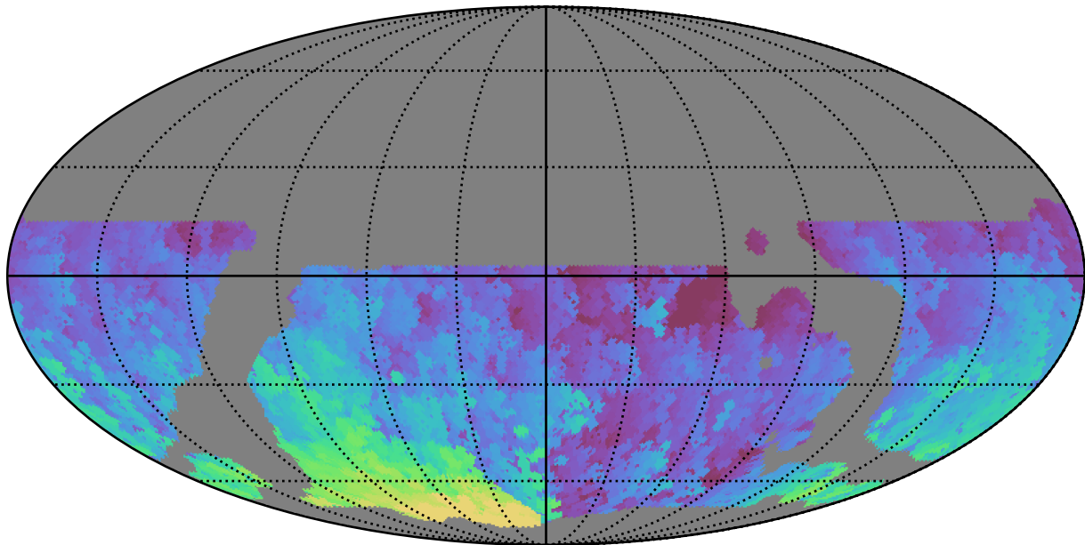
weather_cloudso20v3.4_10yrs WFD g band: Max HA
