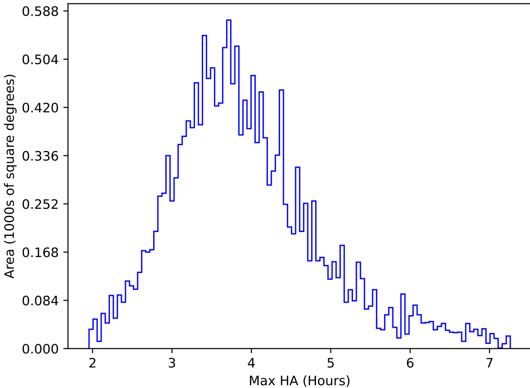
weather_cloudso20v3.4_10yrs WFD g band: Max HA
