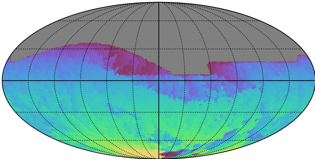
weather_cloudso20v3.4_10yrs All sky z band: Max HA
