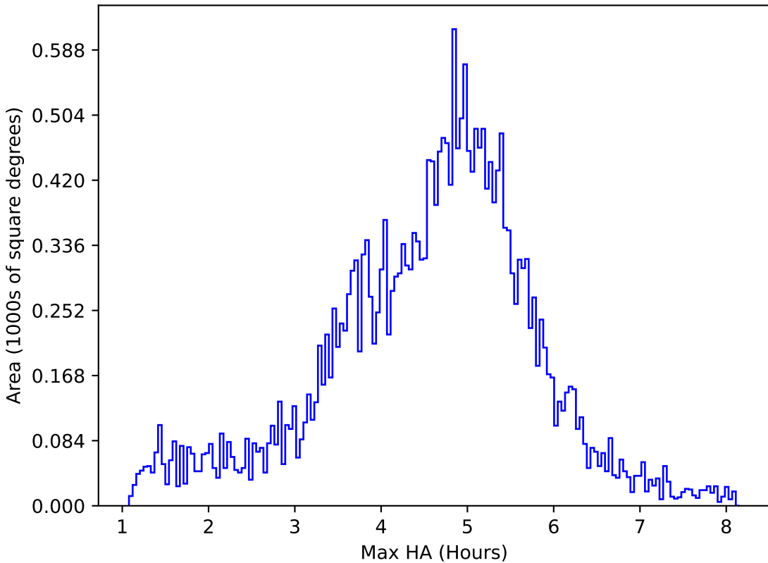
weather_cloudso20v3.4_10yrs All sky z band: Max HA
