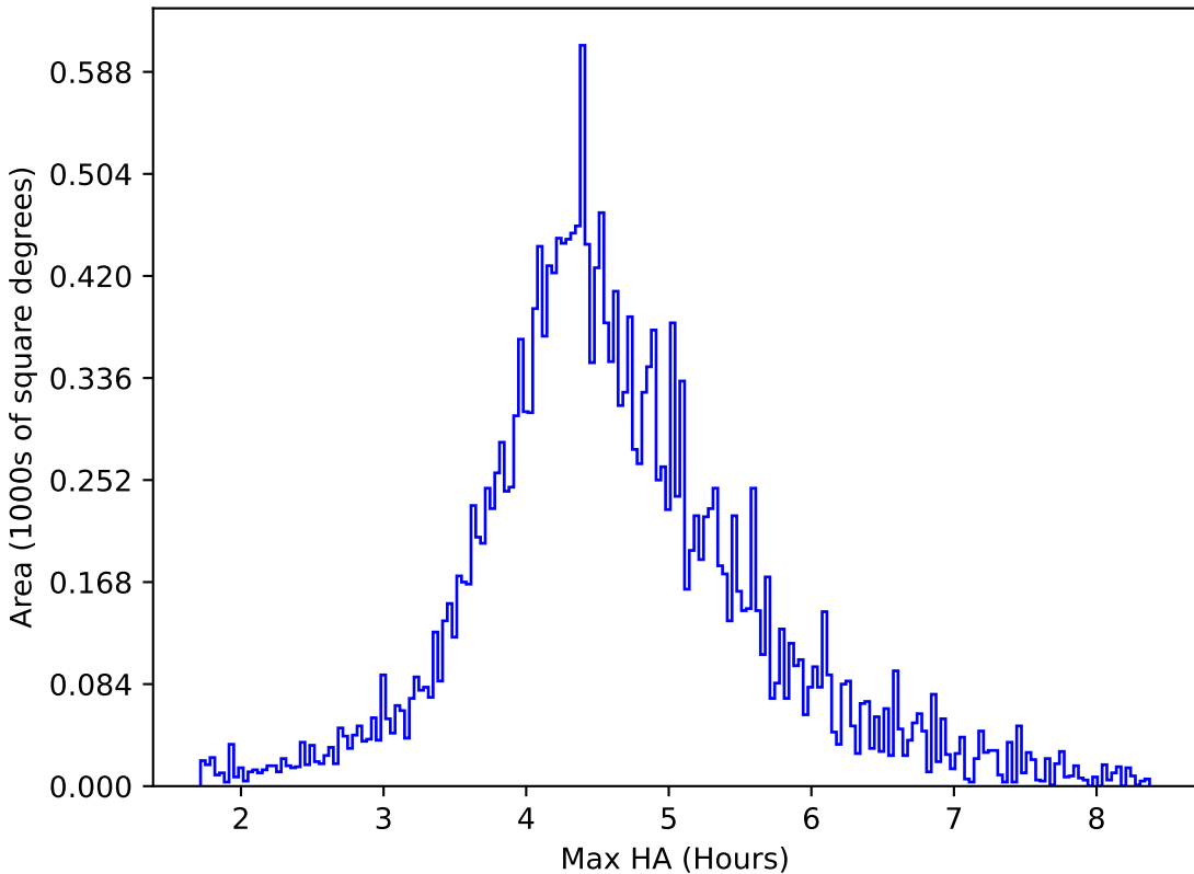
weather_cloudso20v3.4_10yrs All sky y band: Max HA
