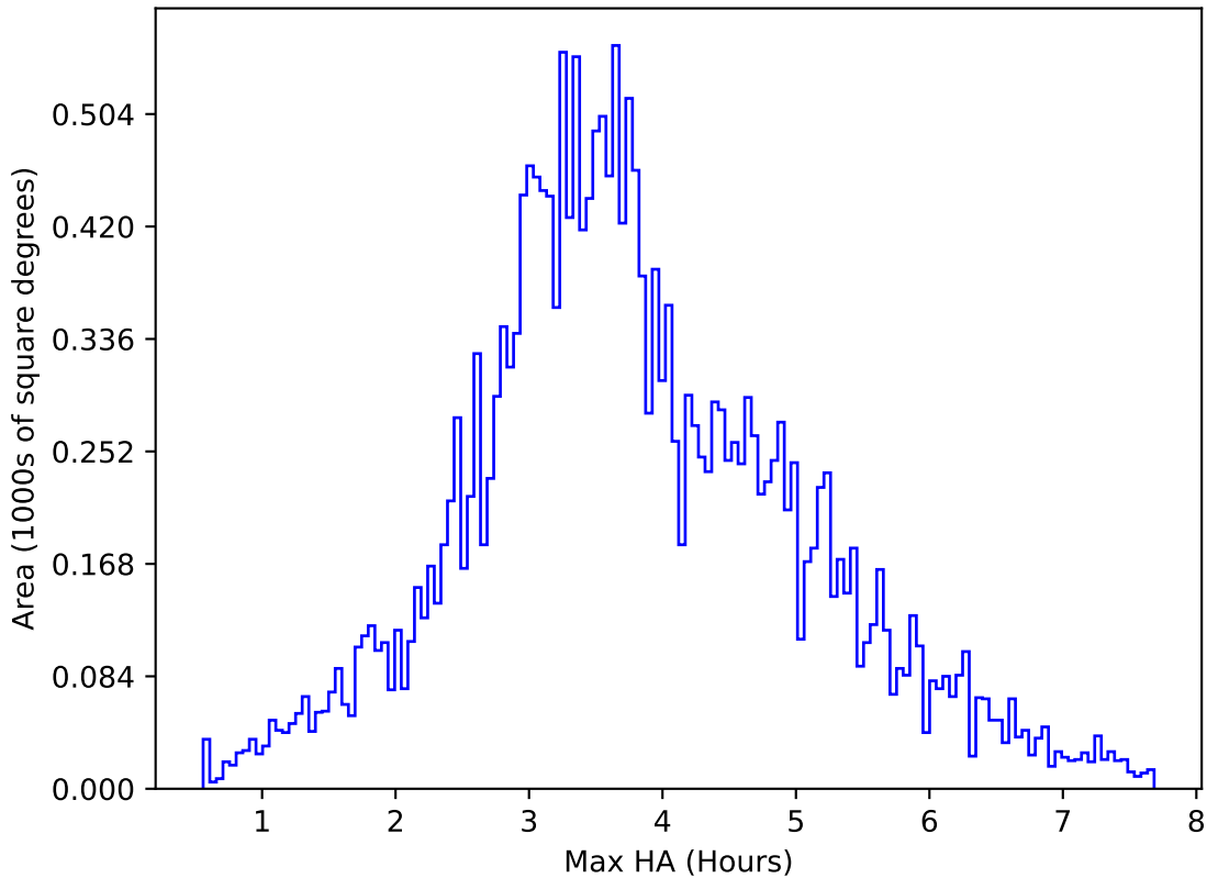
weather_cloudso20v3.4_10yrs All sky u band: Max HA
