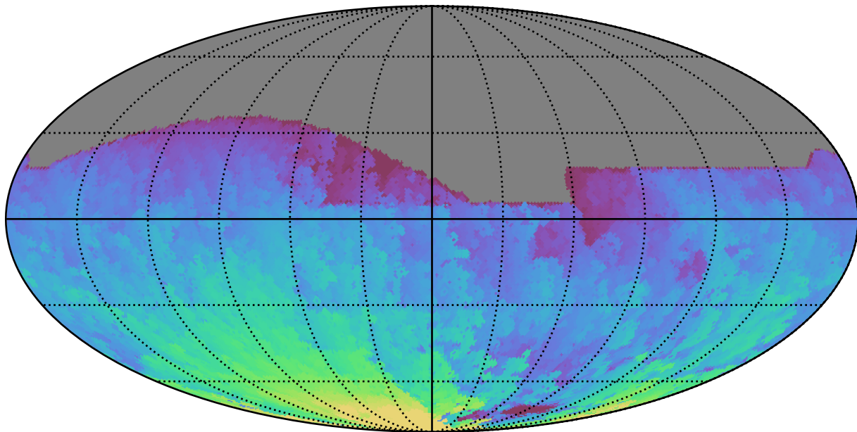
weather_cloudso20v3.4_10yrs All sky r band: Max HA
