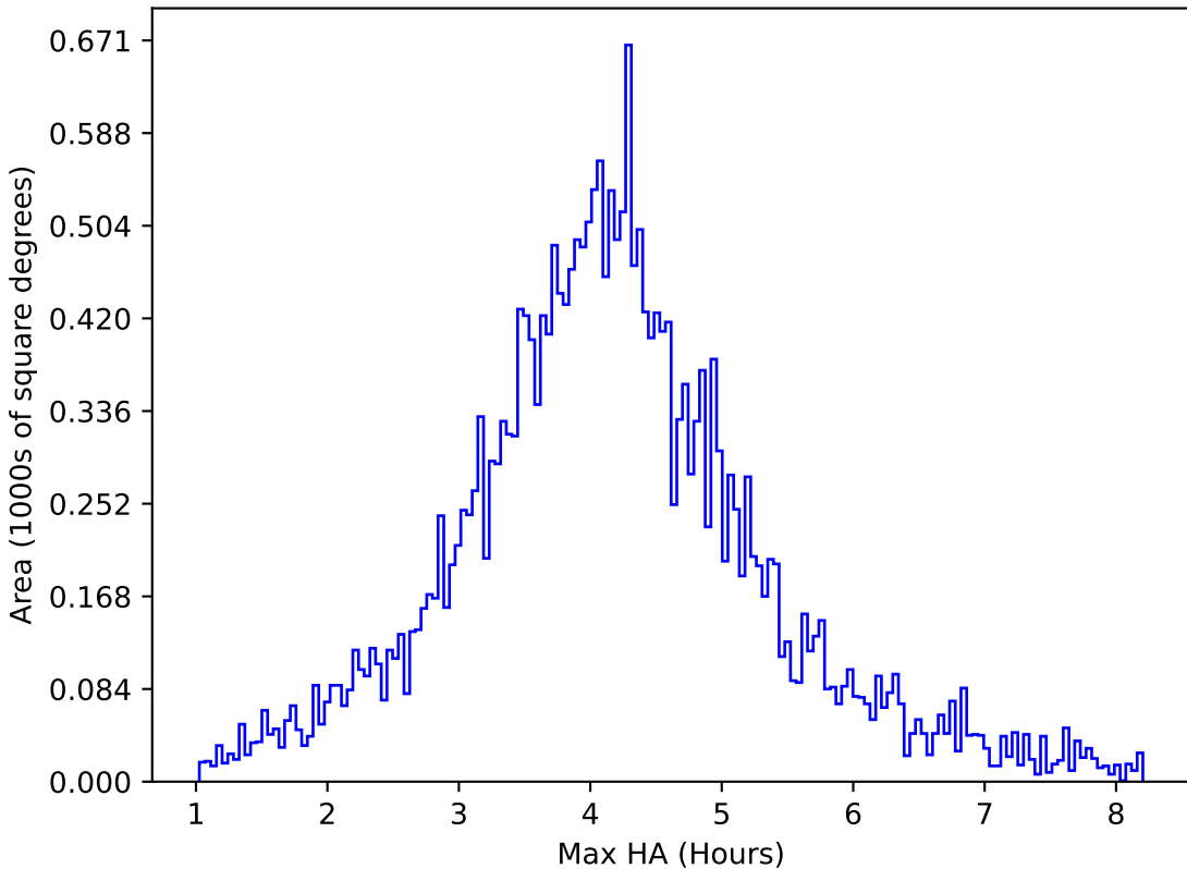
weather_cloudso20v3.4_10yrs All sky r band: Max HA
