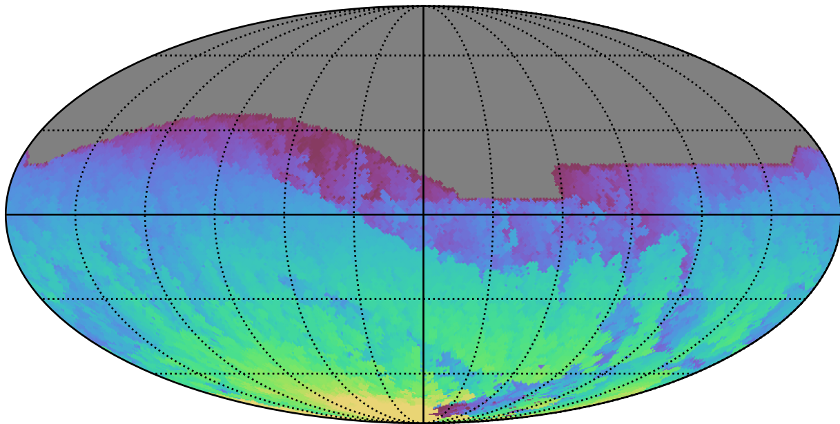
weather_cloudso20v3.4_10yrs All sky i band: Max HA
