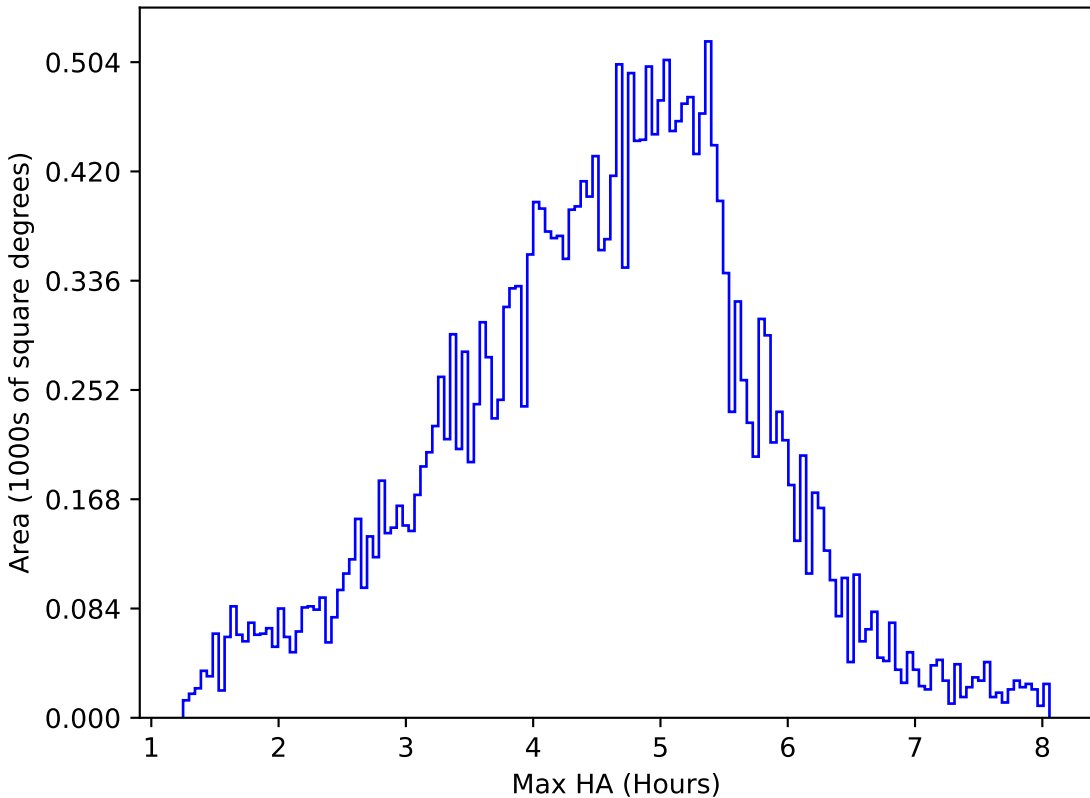
weather_cloudso20v3.4_10yrs All sky i band: Max HA
