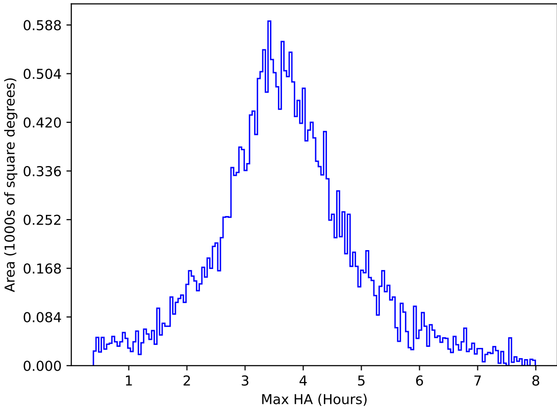
weather_cloudso20v3.4_10yrs All sky g band: Max HA
