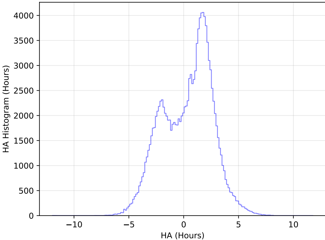
weather_cloudso20v3.4_10yrs WFD u band: HA Histogram
