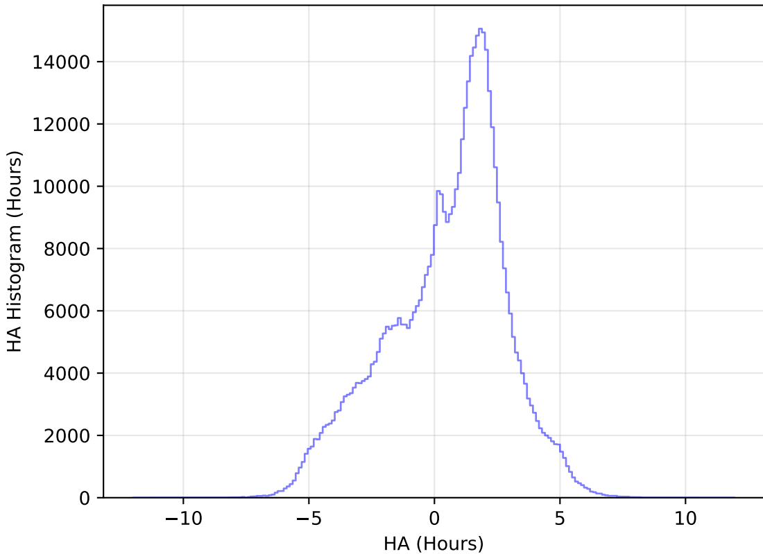
weather_cloudso20v3.4_10yrs WFD i band: HA Histogram
