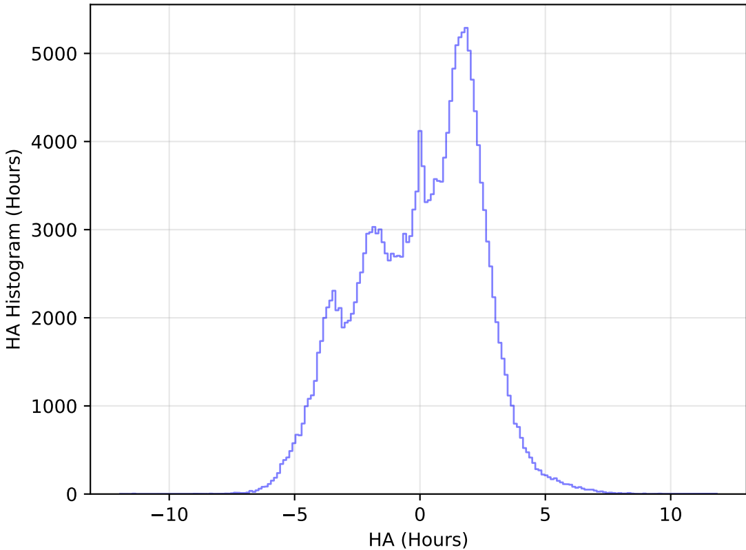
weather_cloudso20v3.4_10yrs WFD g band: HA Histogram
