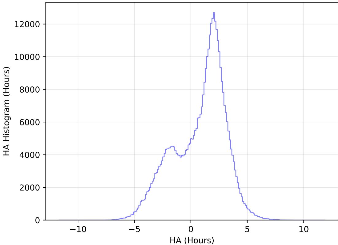
weather_cloudso20v3.4_10yrs All sky y band: HA Histogram
