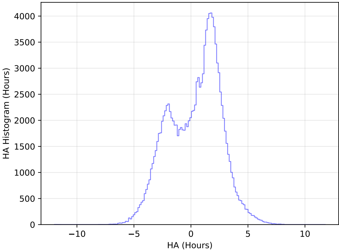
weather_cloudso20v3.4_10yrs All sky u band: HA Histogram
