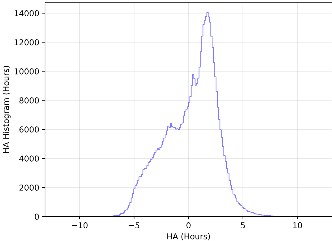
weather_cloudso20v3.4_10yrs All sky r band: HA Histogram
