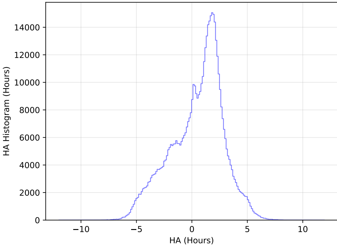
weather_cloudso20v3.4_10yrs All sky i band: HA Histogram
