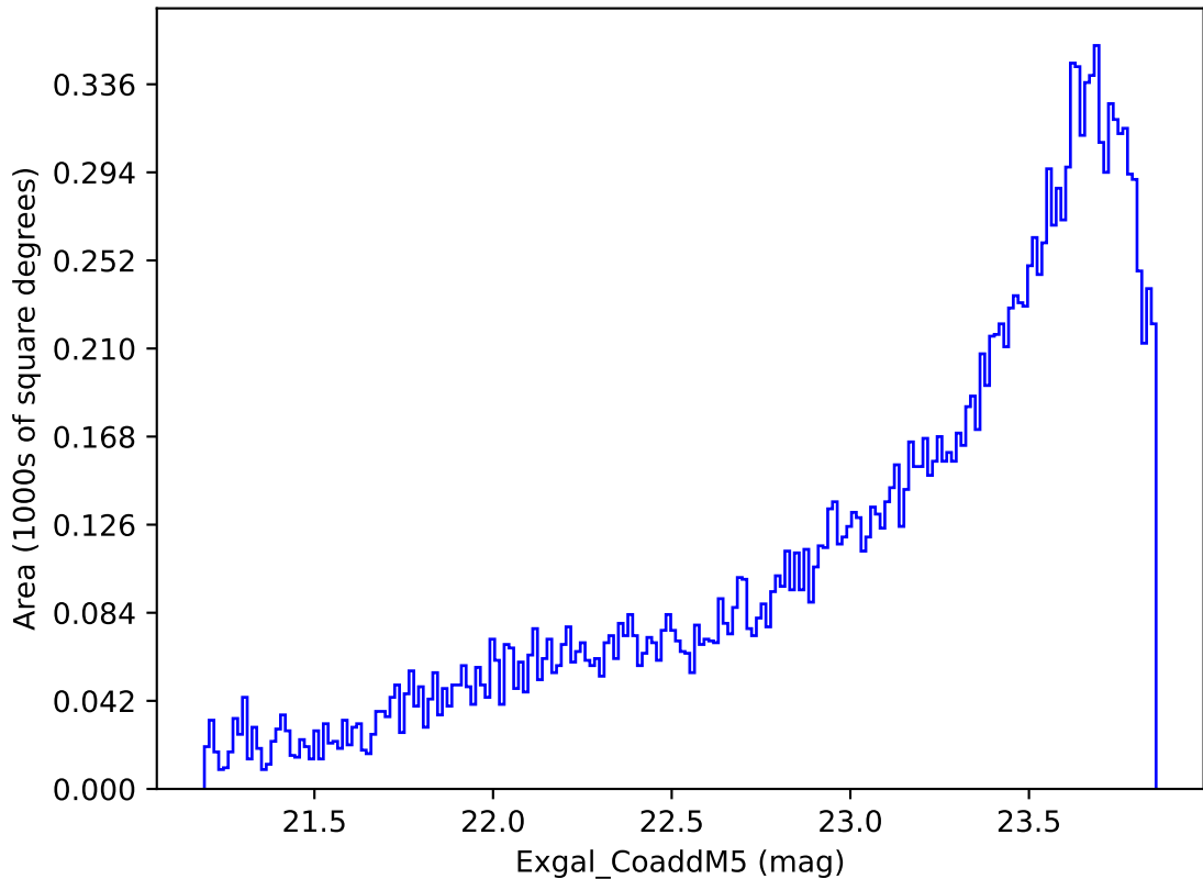
weather_cloudso20v3.4_10yrs Yr 3-4 y band: Exgal_CoaddM5
