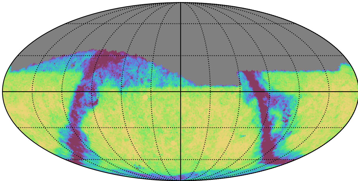
weather_cloudso20v3.4_10yrs Yr 1 z band: Exgal_CoaddM5
