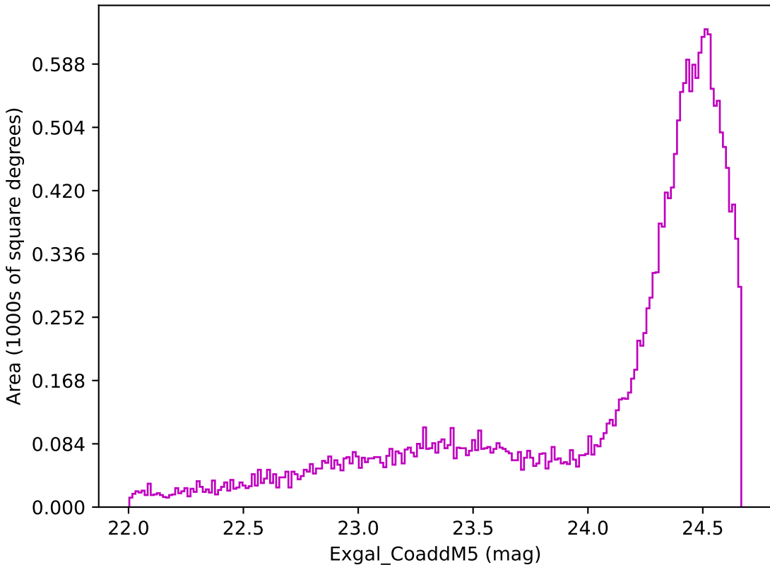
weather_cloudso20v3.4_10yrs Yr 1 z band: Exgal_CoaddM5
