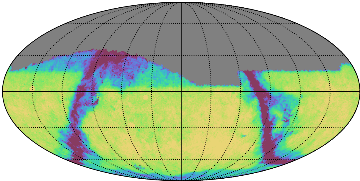
weather_cloudso20v3.4_10yrs Yr 1 i band: Exgal_CoaddM5
