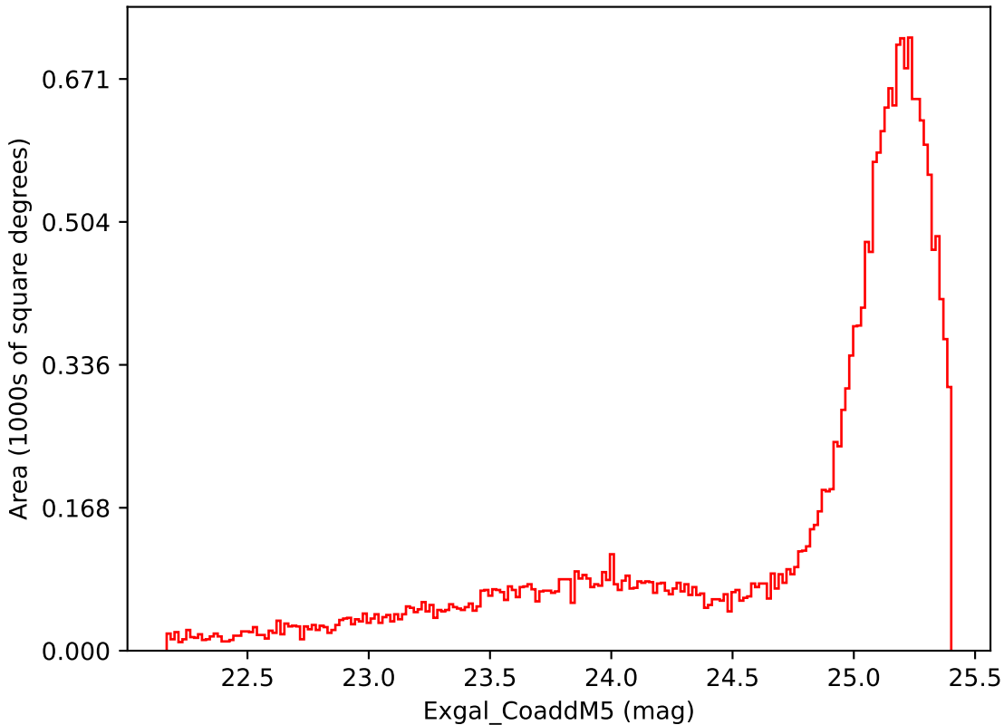
weather_cloudso20v3.4_10yrs Yr 1 i band: Exgal_CoaddM5
