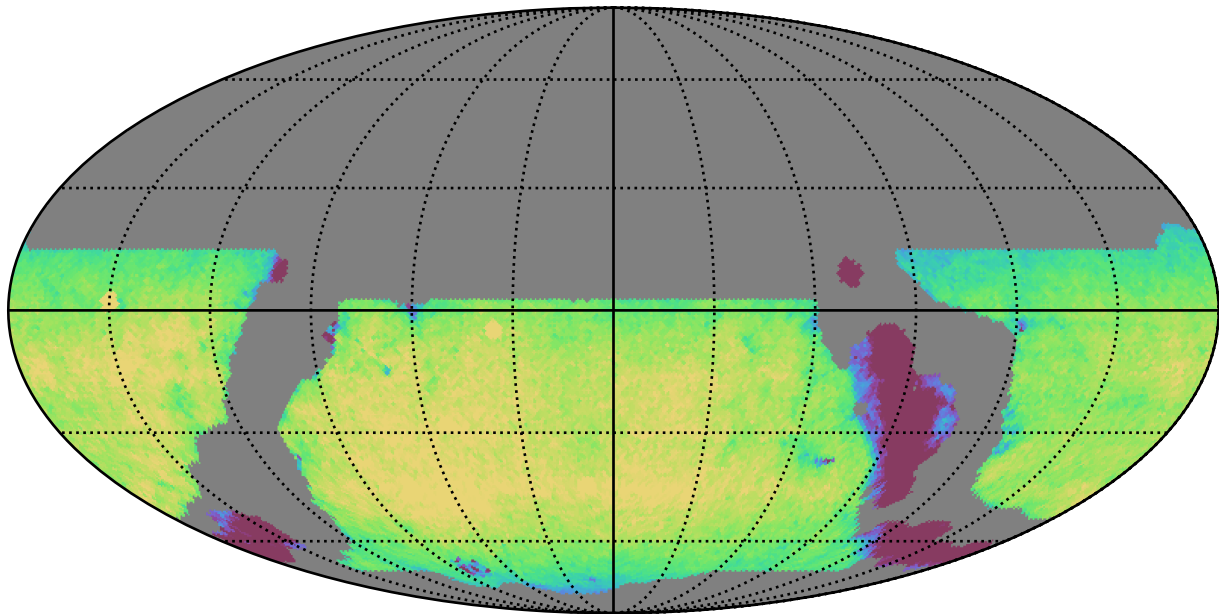
weather_cloudso20v3.4_10yrs WFD y band: Exgal_CoaddM5
