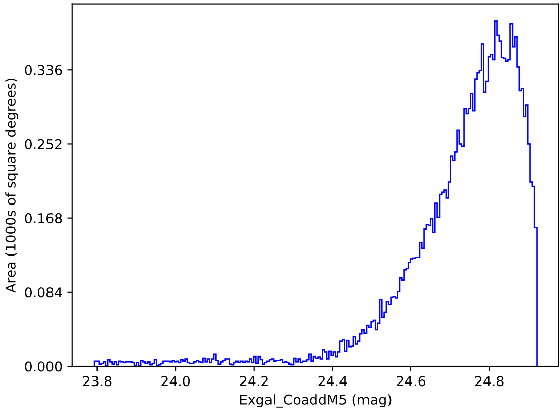
weather_cloudso20v3.4_10yrs WFD y band: Exgal_CoaddM5
