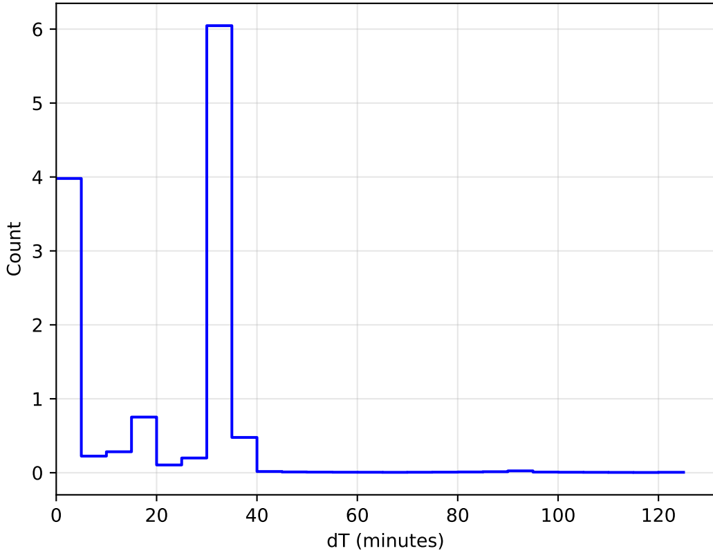
weather_cloudso20v3.4_10yrs WFD: DeltaT Histogram
