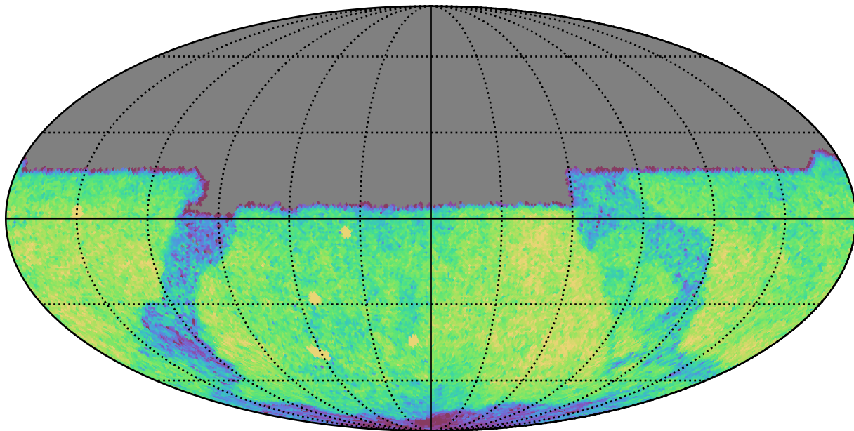
weather_cloudso20v3.4_10yrs Yr 1 y band: CoaddM5
