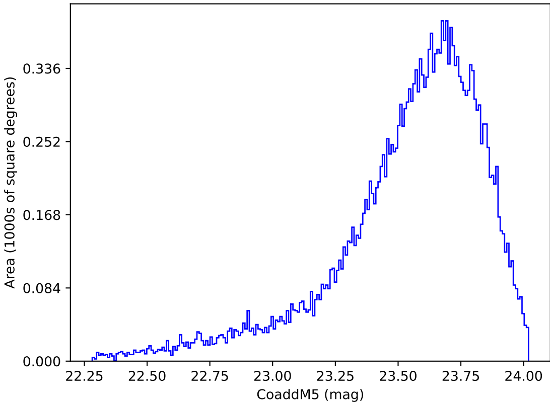
weather_cloudso20v3.4_10yrs Yr 1 y band: CoaddM5
