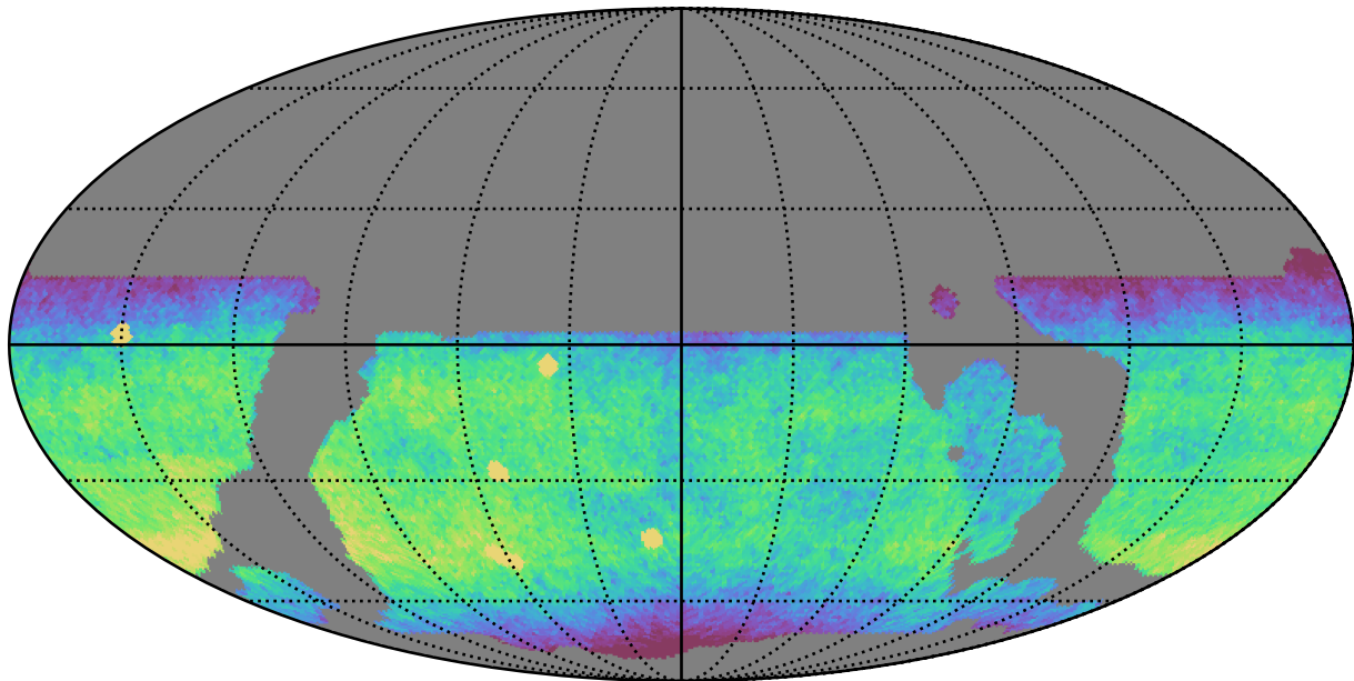
weather_cloudso20v3.4_10yrs WFD z band: CoaddM5
