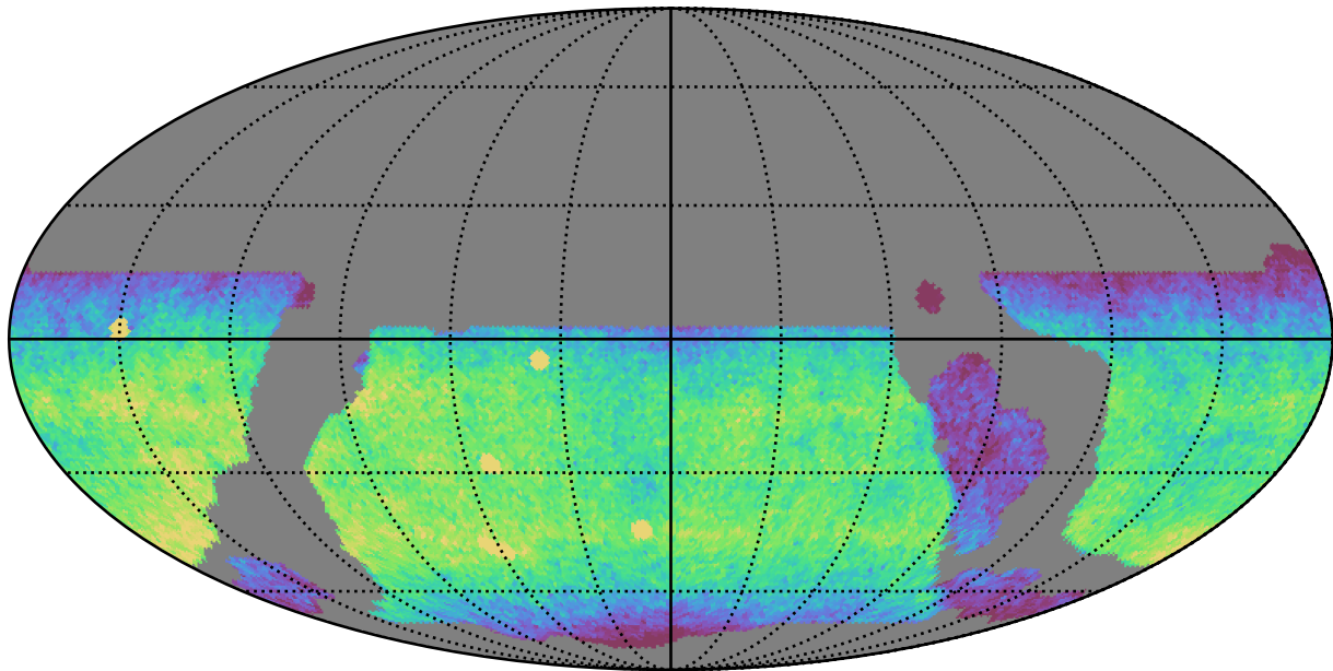
weather_cloudso20v3.4_10yrs WFD y band: CoaddM5
