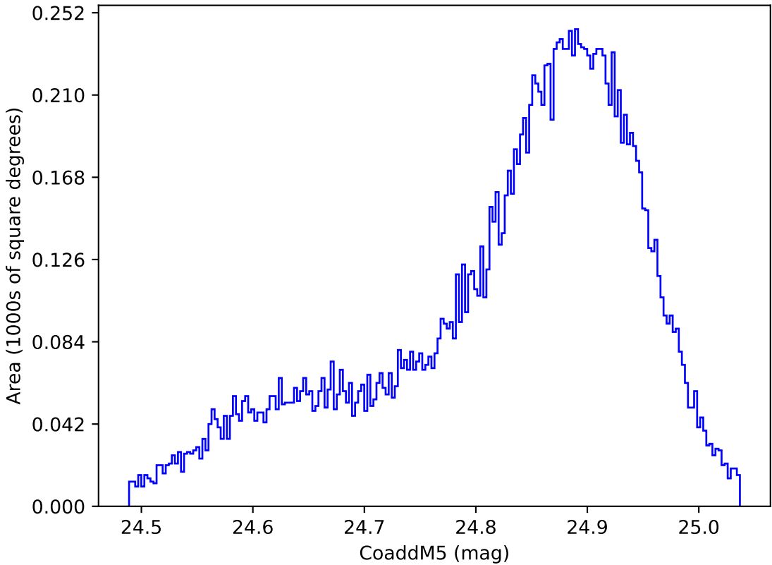
weather_cloudso20v3.4_10yrs WFD y band: CoaddM5
