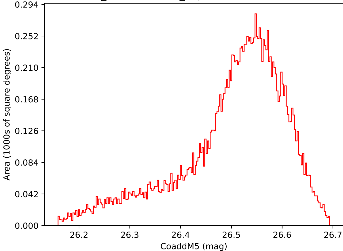
weather_cloudso20v3.4_10yrs WFD i band: CoaddM5
