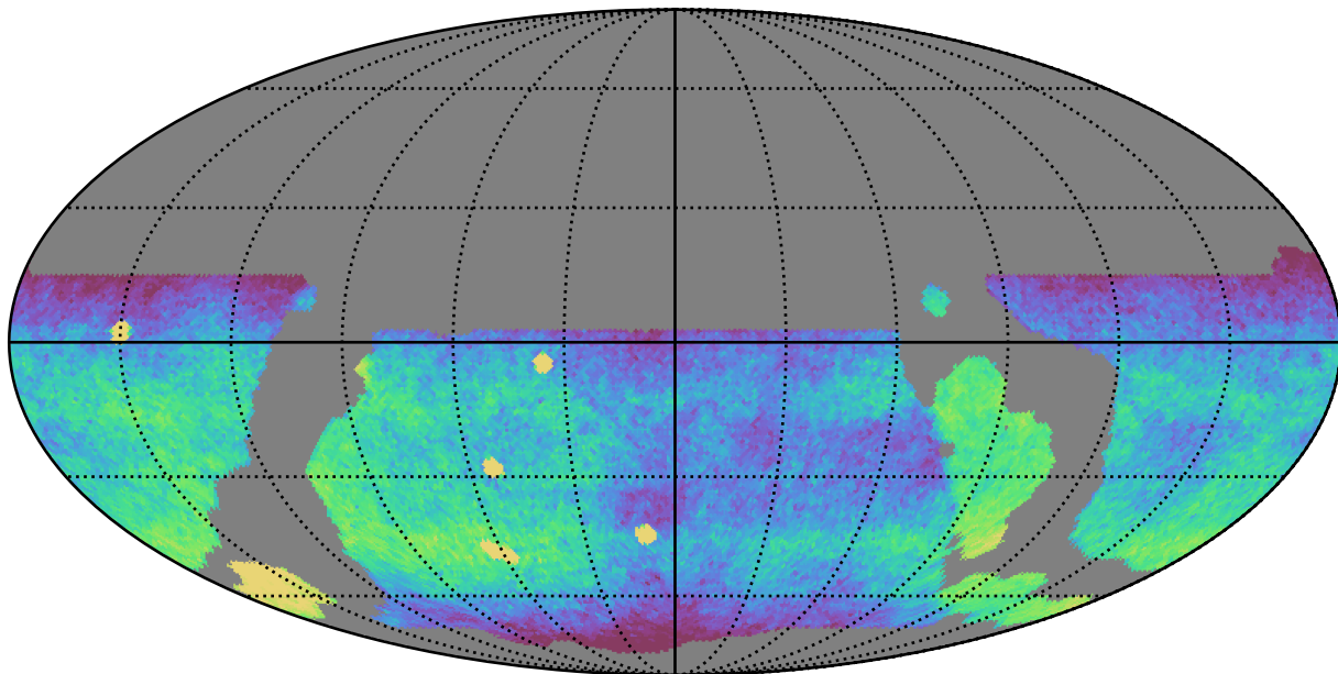
weather_cloudso20v3.4_10yrs WFD g band: CoaddM5
