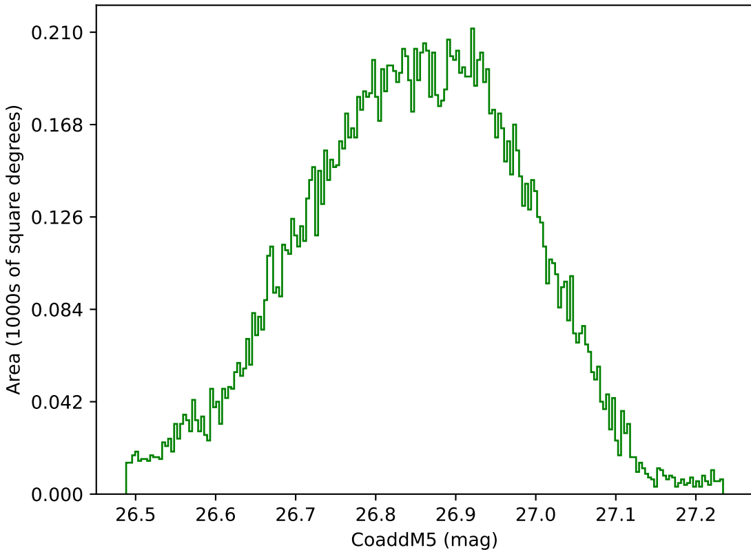
weather_cloudso20v3.4_10yrs WFD g band: CoaddM5
