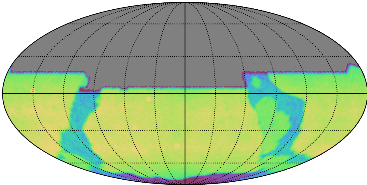
weather_cloudso20v3.4_10yrs All sky y band: CoaddM5
