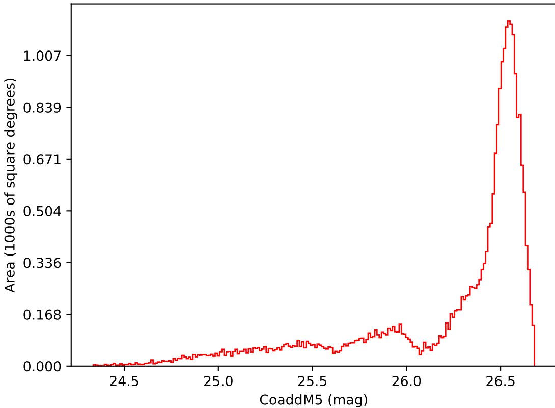
weather_cloudso20v3.4_10yrs All sky i band: CoaddM5
