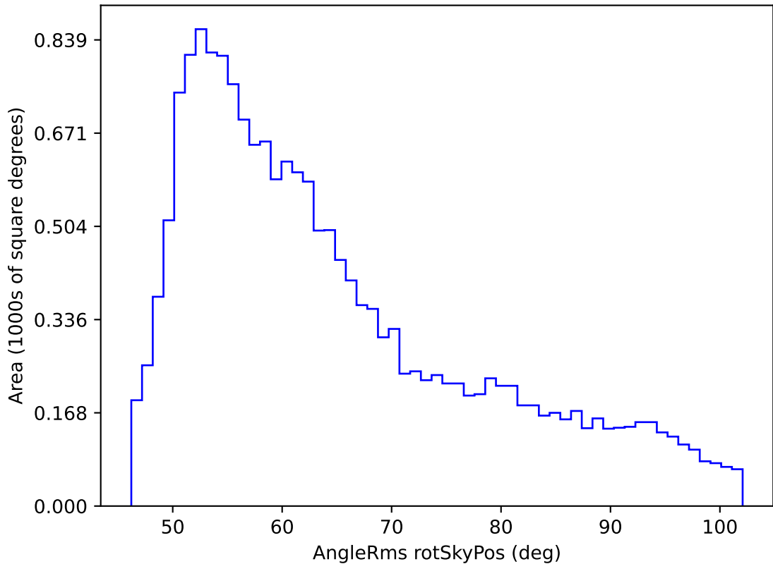
weather_cloudso20v3.4_10yrs WFD y band: AngleRms rotSkyPos
